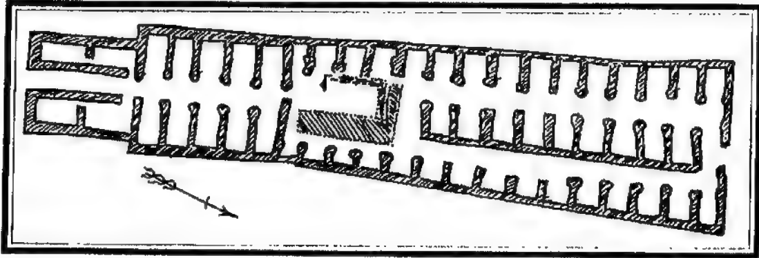
(شكل ٦٦) مسقط أفقى للمقبرة فV فى أبيدوس.
